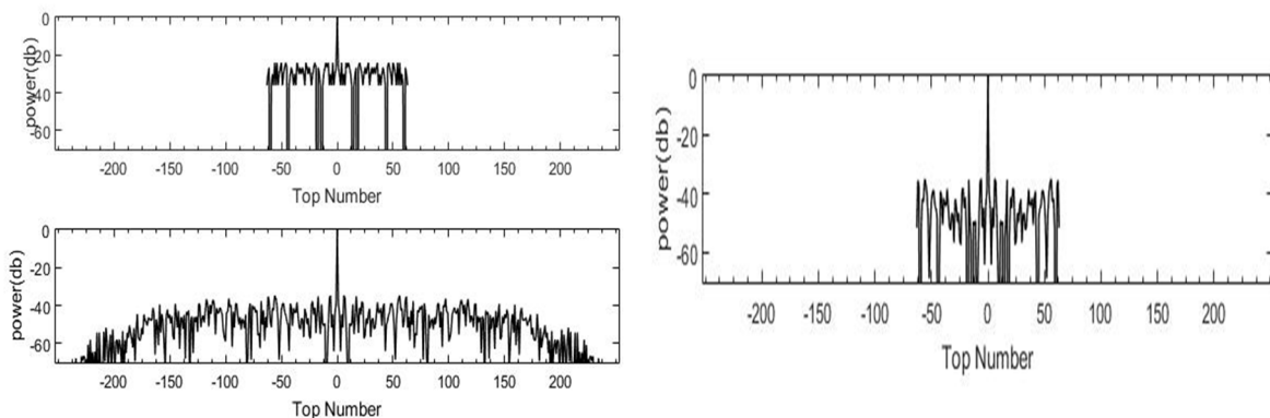
شکل (۴) بالا چپ خروجی: فیلتر منطبق و پایین چپ فیلتر (R-G-3) و شکل راست مینیمم گیری با رابطه (۲۰) برای کد ۶۴ تایی
