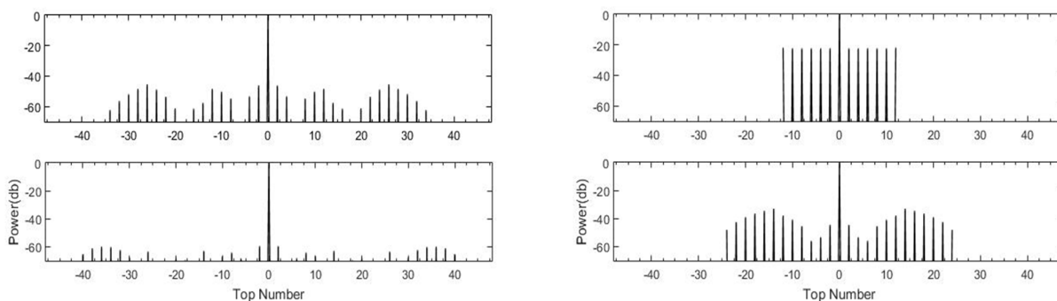
شکل (۱) خروجی: فیلتر منطبق MF (بالا راست) فیلتر (R-G-1) (پایین راست) فیلتر (R-G-2) (بالا چپ) و فیلتر (R-G-3) (پایین چپ) برای بارکر
