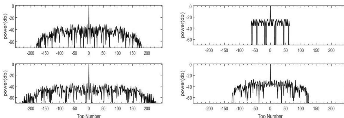
شکل (۲) خروجی: فیلتر منطبق (بالا راست) و فیلتر (R-G-1) (پایین راست) و فیلتر (R-G-2) (بالا چپ) و فیلتر (R-G-3) (پایین چپ) برای کد ۶۴
