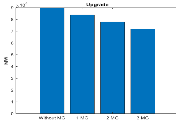
شکل ۴. مقدار ظرفیت توسعه شبکه انتقال
