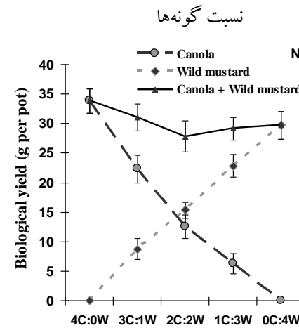
شکل ۱- عملکرد بیولوژیک کلزا (C) و خردل وحشی (W) و مجموع تولید دو گونه در گلدان در نسبت‌های مخلوط (N1=۰/۷۵، N2=۱، N3=۱/۲۵، N4=۱/۵۰ گرم نیتروژن در گلدان).
