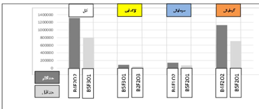
شکل ۸- نتایج شبیه‌سازی حداکثر و حداقل مصرف انرژی کل (گرمایش، سرمایش و روشنایی) به ازای کیلووات ساعت بر متر مربع
