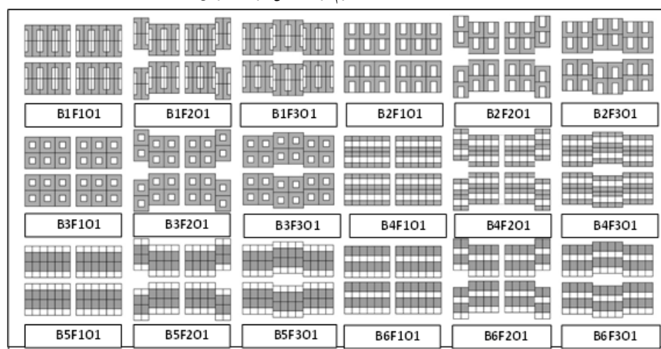
شکل ۱۱- ریخت گونه شناسی مدل‌های تحلیلی برای شبیه‌سازی مصرف انرژی در جهت استقرار (O1). قابل ذکر است که این مدل‌ها در سه جهت دیگر شناسایی شده تغییر یافته و جمعاً ۷۲ شبیه‌سازی مصرف انرژی انجام گرفته است. Source: Research findings, 2018
