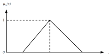
شکل ۳- عملکرد عضویت یک عدد فازی سه وجهی \tilde{M} = (l, m, u)
