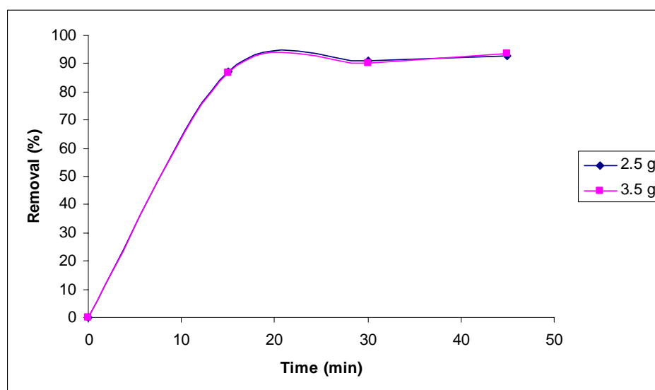
نمودار ۳- بررسی اثر زمان بر درصد جذب در \text{pH}=7 در دمای آزمایشگاه
