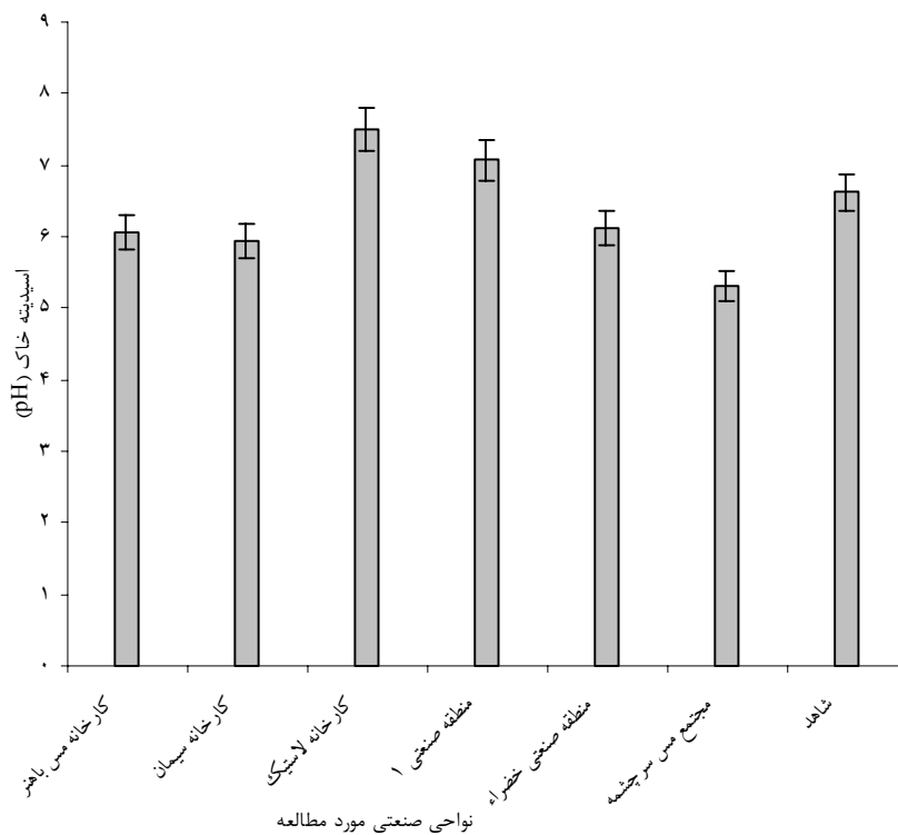
نمودار ۲- مقایسه میانگین اسیدیته خاک (pH) در برخی نواحی صنعتی مهم استان کرمان
