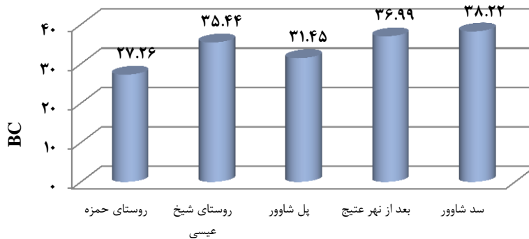
نمودار ۳- شاخص کیفی BCWQI Figure 3. BC Water Quality Index
