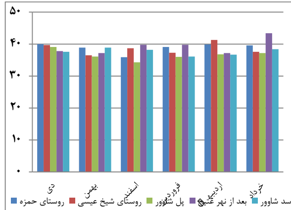
نمودار ۱- شاخص کیفی NSFQI Figure 1. NSF Water Quality Index
