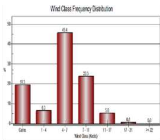
شکل ۴- طبقه بندی سرعت باد در ماه ژوئن در ایستگاه اراک Figure 4. Classification of wind speed in June at Arak station
