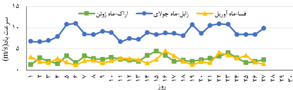
شکل ۱- نمودار تغییرات سرعت باد در منطقه مورد مطالعه Figure 1. The plot of wind speed in the studied area
