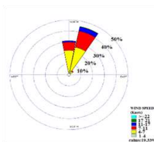
شکل ۳- گلباد مربوط به ماه ژوئن در ایستگاه اراک Figure 3. Windrose in June at Arak station
