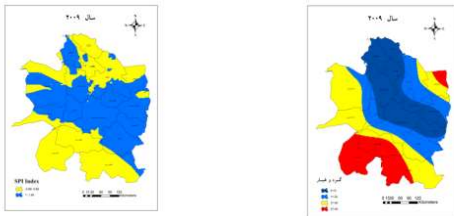
شکل ۸- نقشه‌های پهنه‌بندی گرد و غبار و شاخص خشک‌سالی SPI برای سال ۲۰۰۹ Figure 8. Zoning maps dust and SPI drought index for 2009
