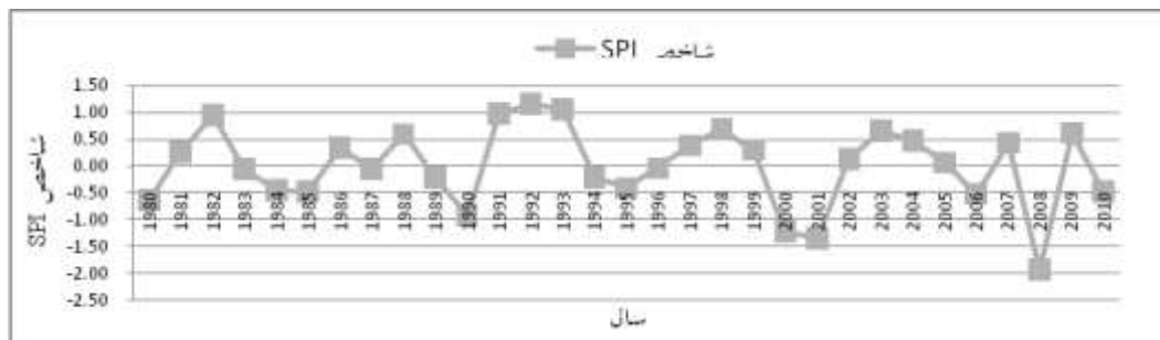
شکل ۲- تغییرات شاخص خشک‌سالی SPI در دوره مورد مطالعه
