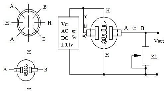
شکل ۲- مدار بندی (راست) و نحوه قرارگیری پایه‌های یکی از حسگرها (چپ)
