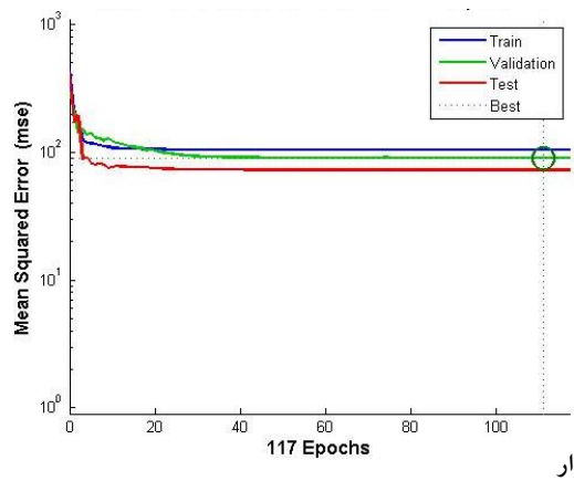
شکل ۴- تغییرات تابع هدف (میانگین مربعات خطا) برای داده‌های آموزش، اعتبارسنجی و آزمون
