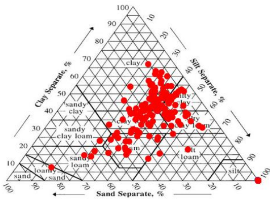
شکل ۲- توزیع کلاس بافتی خاک‌های منطقه مورد مطالعه
