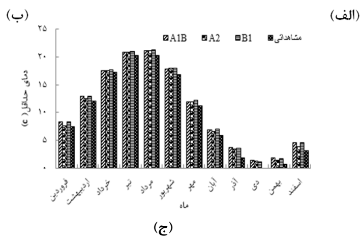
شکل ۳. میانگین‌های ماهانه مشاهداتی (۱۹۸۵-۲۰۱۰) و شبیه‌سازی شده (الف) بارش، (ب) دمای حداکثر و (ج) دمای حداقل در دوره آتی (۲۰۱۱-۲۰۳۰) تحت سناریوهای مختلف
