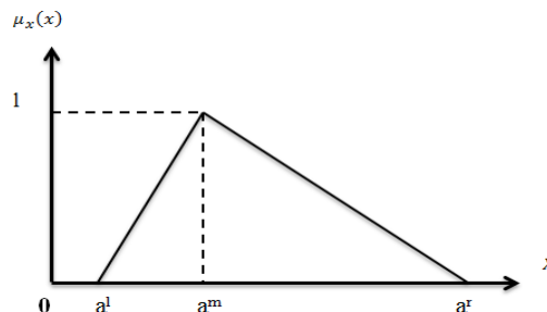
نگاره ۱- نمایش عدد فازی مثلثی
