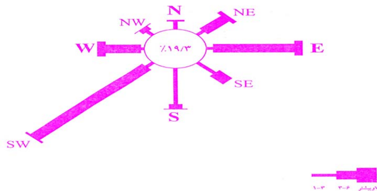
شکل شماره ۸: نمودار گلباد سینوپتیک بندر لنگه، ۱۹۹۵-۱۹۸۲ م
