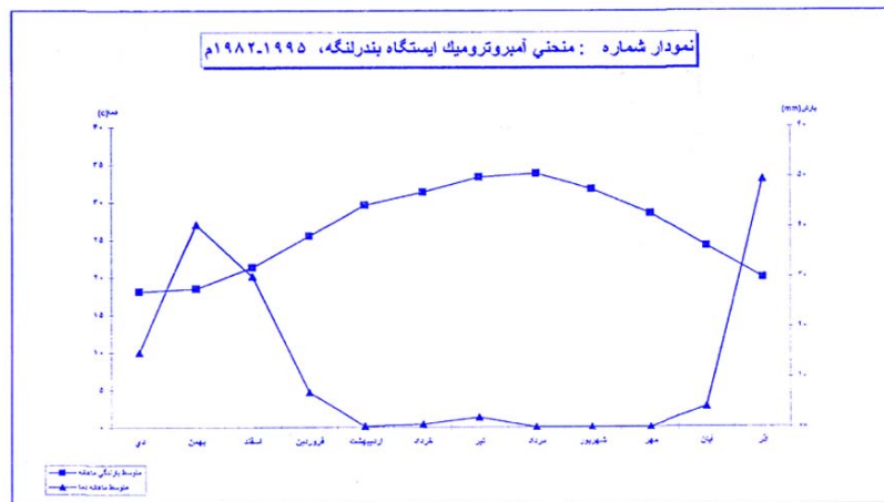
شکل شماره ۷: نمودار منحنی آمپروترومیک ایستگاه سینوپتیک بندر لنگه، ۱۹۹۵-۱۹۸۲م
