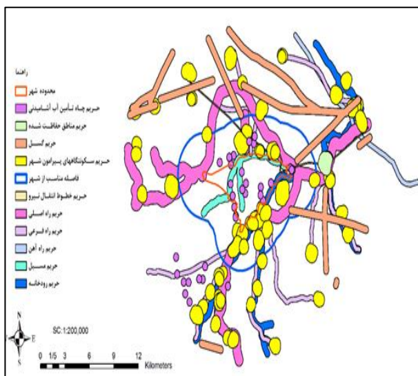
شکل ۹: حرائم حذف شده از مکان‌یابی تصفیه‌خانه فاضلاب
