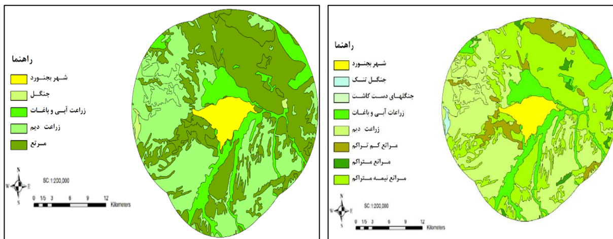
شکل ۶: پوشش گیاهی محدوده مطالعه
