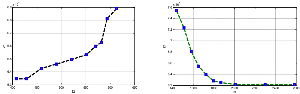
شکل ۴: نمودار جبهه پارتو هدف اقتصادی (Z ۱ ) نسبت به هدف اجتماعی (Z ۲ ) و هدف زیست‌محیطی (Z ۳ )
