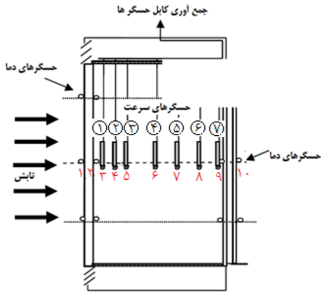
شکل ۲. مقطع نمای دو پوسته آزمایشگاهی می و همکاران و محل تعبیه حسگرهای حرارتی و سرعت سنج (Mei et al., 2007) Figure 2. Cross-sectional view of double skin facade of May et al. test and the location of thermal and velocity sensors (Mei et al., 2007)
