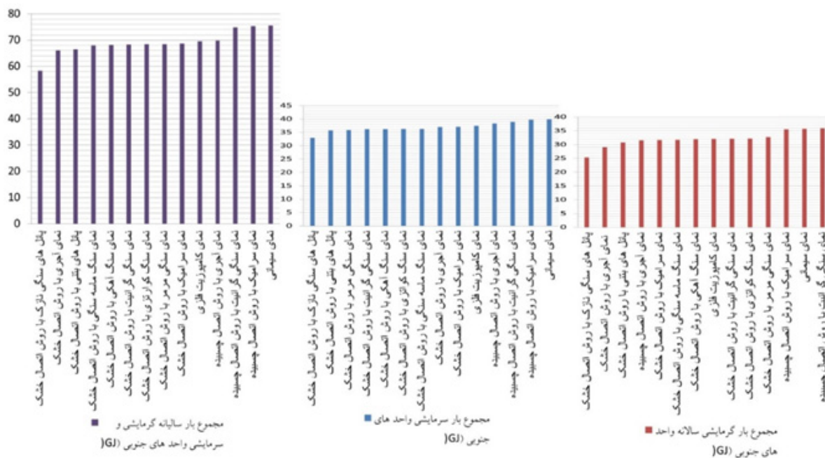
شکل ۴. مقایسه انرژی مصرفی در ساختمان‌های رو به جنوب با انواع مختلف نماسازی. Figure 4. The comparison of energy consumption in south-facing buildings with different facades.
