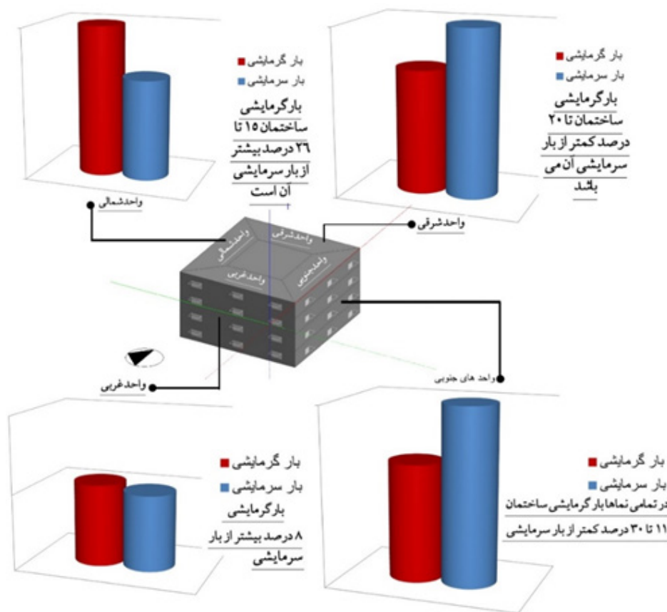
شکل ۸. مقایسه نسبت بار گرمایشی به سرمایشی در نماهای مختلف.
