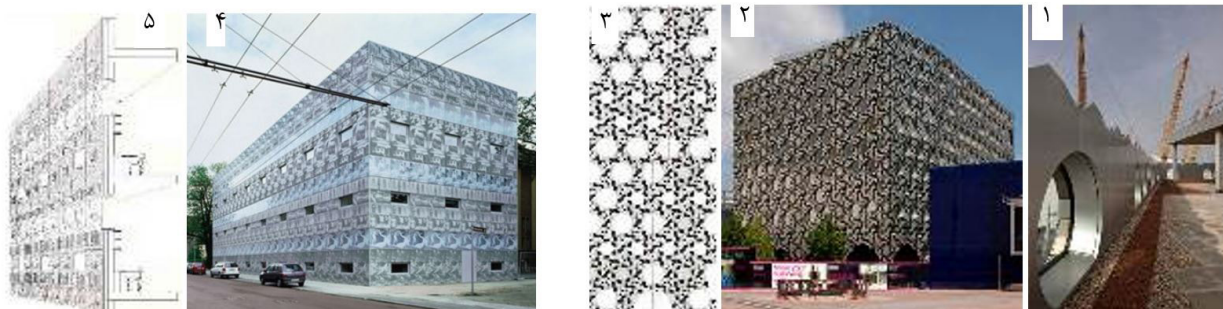
شکل ۵. ۱، ۲، ۳: تلاقی گشودگی با خطوط لبه بام، پنهان شدن ستون در پشت‌نما، نشان از عدم هماهنگی پوسته تزئینی با ساختار سازه و عملکرد و مقیاس بنا دارد (Foreign Office Architects, 2009). ۴، ۵: کتابخانه مدرسه فنی ابرسوال (Picon, 2014)، تکرار الگوی ثابت در یک شبکه، بافتی بی‌تفاوت نسبت به ساختار سازه‌ای و عملکرد و نیز مقیاس واقعی بنا به وجود آورده است.
