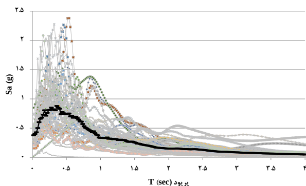
شکل ۱- طیف پاسخ شتاب الاستیک مربوط به ۴۴ رکورد منتخب و طیف میانه آنها
