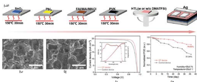
شکل ۸. (الف) طرح واره ای از ساخت سلول پروسکایتی در شرایط با و بدون استفاده از DMATFSI. تصویر SEM از سطح لایه پروسکایت پس از حذف (ب) LiTFSI و (ج) دوپ همزمان LiTFSI و DMATFSI. بازدهی (د) و پایداری (ه)
