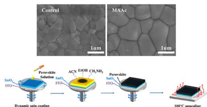
شکل ۵. دستیابی به بازدهی بالای ۱۹ درصد و پایداری عملکرد ۸۰ درصدی در مدت زمان ۵۰۰ ساعت تحت رطوبت ۴۰ درصد برای سلول‌های پروسکایتی حاوی MAAc ساخته شده با روش لایه‌نشانی چرخشی تک مرحله‌ای [۳۳].
