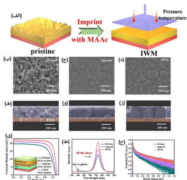
شکل ۷. (الف) طرح واره ای از تغییرات ریزساختار بعد از تیمار IWM. تصویر SEM از سطح و مقطع لایه های پروسکایت (ب، ه، ج، و)، Imprint، (د، ز)، IWM. (ح) طیف TRPL و (ط) PL لایه های پروسکایت مذکور، (ی) منحنی چگالی جریان - ولتاژ سلول های پروسکایتی حاصل که افزایش حدود ۵ درصد در بازدهی از طریق IWM مشهود است [۴۸].
