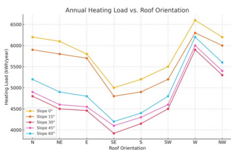
شکل ۴. بار گرمایشی سالانه سناریوها (مأخذ: نگارندگان)
