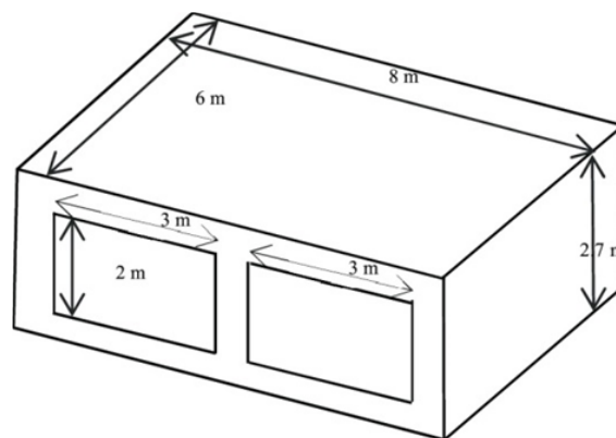
شکل ۱. نمونه ساختمانی پایه (مأخذ: Mirabi & Akrami Abarghuie, 2021) Figure 1. Sample of basic building (Source: Mirabi & Akrami Abarghuie, 2021)
