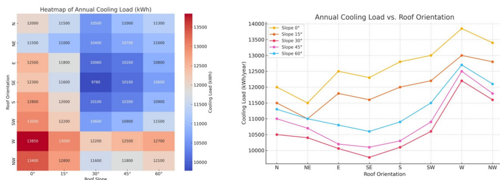
شکل ۳. بار سرمایشی سالانه سناریوها (مأخذ: نگارندگان) Figure 3. Annual cooling load of scenarios (Source: Authors)
