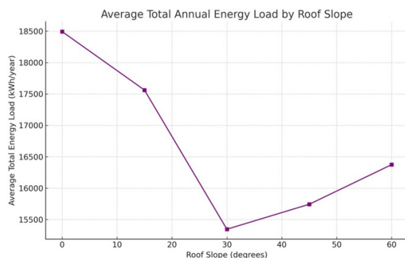
شکل ۵. متوسط بار انرژی سالانه سناریوها براساس زاویه شیب بام (مأخذ: نگارندگان)
