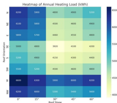
شکل ۴. بار گرمایشی سالانه سناریوها (مأخذ: نگارندگان)
