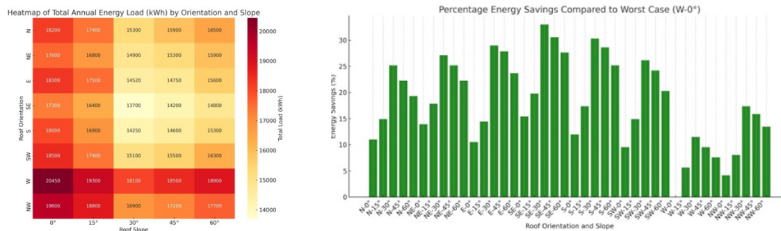
شکل ۷. درصد کاهش مصرف انرژی هر سناریو (مأخذ: نگارندگان) Figure 7. Percentage reduction in energy consumption for each scenario (Source: Authors)
