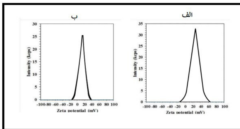
شکل ۲. نمودار پتانسیل زتا نمونه ها: الف: پتانسیل زتای نانوکیتوزان (+20/5) ، ب: پتانسیل زتای نانوکیتوزان حامل عصاره هیدروالکلی دانه گرده گل (+19/4) میلی ولت
