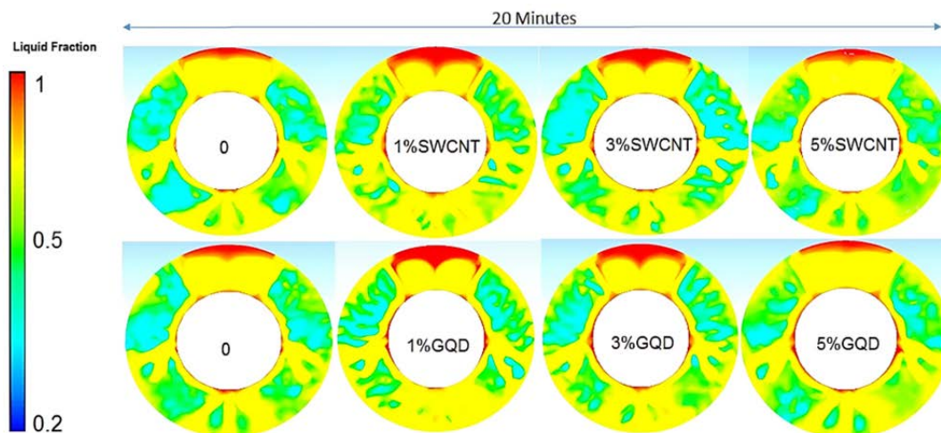
شکل ۳ اثرهای مقدارهای متفاوت نانوذره‌های GQD و SWCNTs بر فرایند ذوب مواد تغییرفازدهنده [۳۳] (دارای مجوز از ناشر مربوط)
