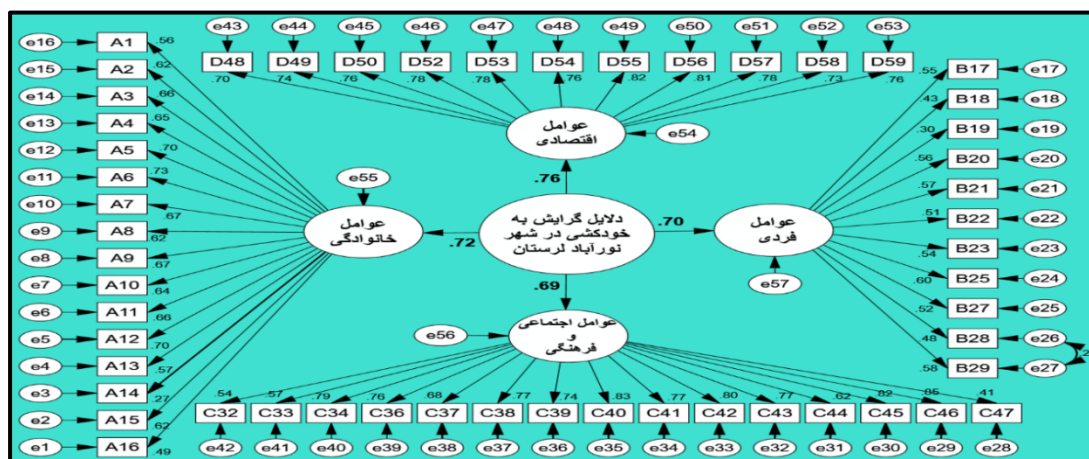
شکل ۴. مدل تحلیلی عاملی تأییدی در حالت برآورد ضرایب استاندارد Source: Research findings, 2023
