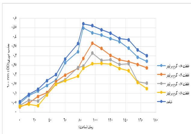
شکل ۲: منحنی رشد باسیلوس مجاونسیس در غلظت‌های مختلف فناترن.
