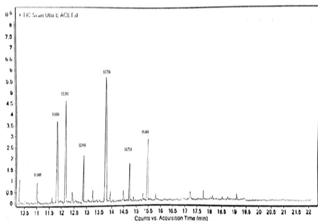
شکل ۳: نمودار کروماتوگرام تجزیه فنانترن توسط باکتری باسیلوس مجاونسیس.
