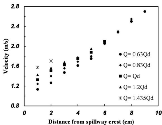
شکل ۱۰- تغییرات سرعت جریان در نمونه سرریز
