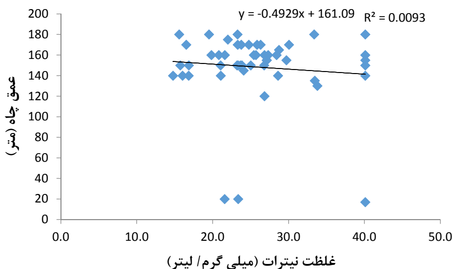
شکل ۴- همبستگی بین غلظت نیترات در آب زیرزمینی با عمق چاه در دشت سرجهان
