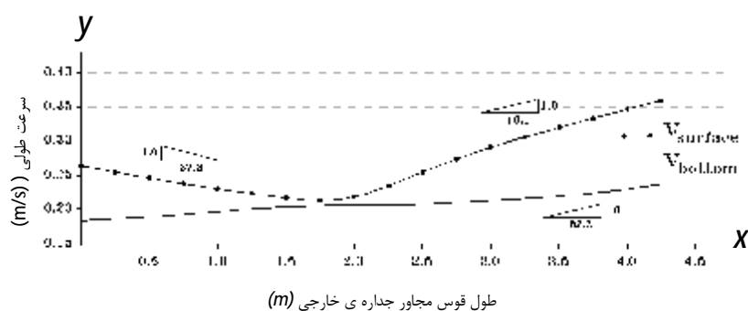
شکل 9. سرعت طولی مجاور جداره ی خارجی در قوس 4.
