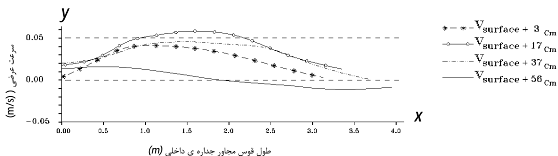
شکل 13. سرعت عرضی مجاور لایه ی سطح در قوس 3.
