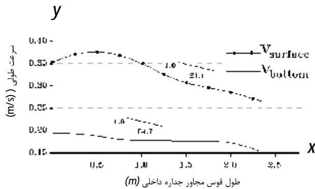
شکل 12. سرعت طولی مجاور جداره‌ی داخلی در قوس 3.
