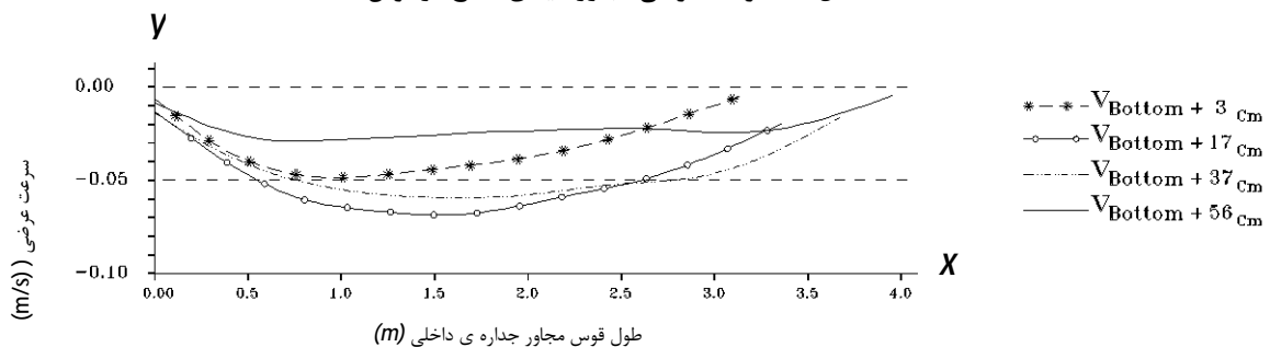
شکل 14. سرعت عرضی مجاور لایه ی کف در قوس 3.
