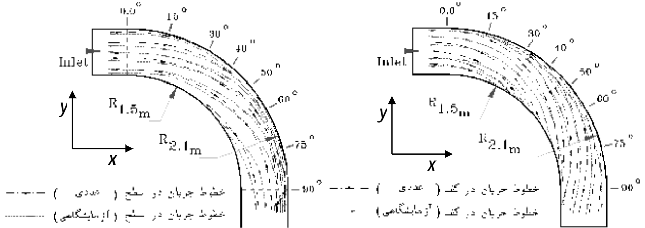
شکل 4. خطوط جریان در قوس 3.
