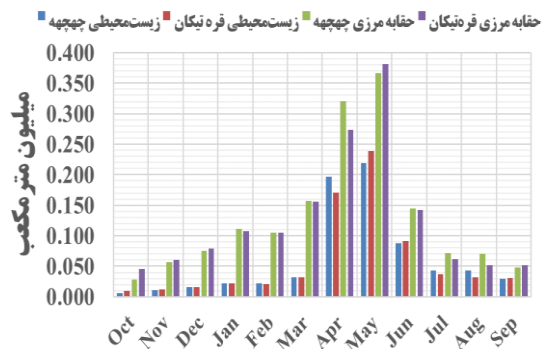
(د) میزان حجم جریان تامین شده حقابه زیست محیطی رودخانه ها و پروتکل مرزی مشترک پس از احداث سد
