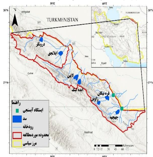
شکل ۱- موقعیت محدوده مورد مطالعه به همراه جانمایی ایستگاه‌های هیدرومتری منتخب و سدهای حوضه‌آبریز
