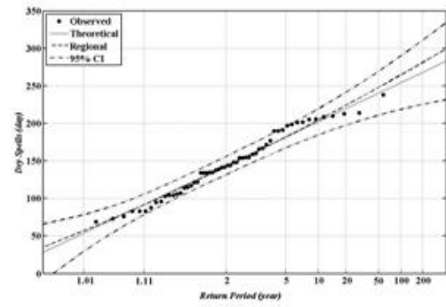
شکل ۱۰- تابع توزیع چگالی احتمال تجمعی دوره‌های بدون بارش برای ایستگاه کرمان (گروه ۱).
