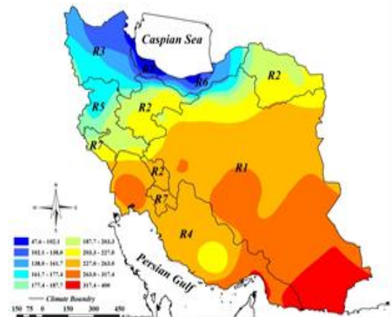
شکل ۲۴- نقشه ی حداکثر سالانه ی روز های بدون بارندگی در دوره ی برگشت ۵۰ ساله. شکل ۲۵- نقشه ی حداکثر سالانه ی روز های بدون بارندگی در دوره ی برگشت ۱۰۰ ساله.
