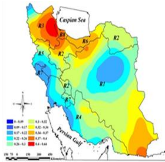
شکل ۳- ضریب تغییرات حداکثر تعداد روزهای بدون بارندگی ایران.
