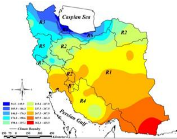
شکل ۲۴- نقشه ی حداکثر سالانه ی روز های بدون بارندگی در دوره ی برگشت ۵۰ ساله. شکل ۲۵- نقشه ی حداکثر سالانه ی روز های بدون بارندگی در دوره ی برگشت ۱۰۰ ساله.
