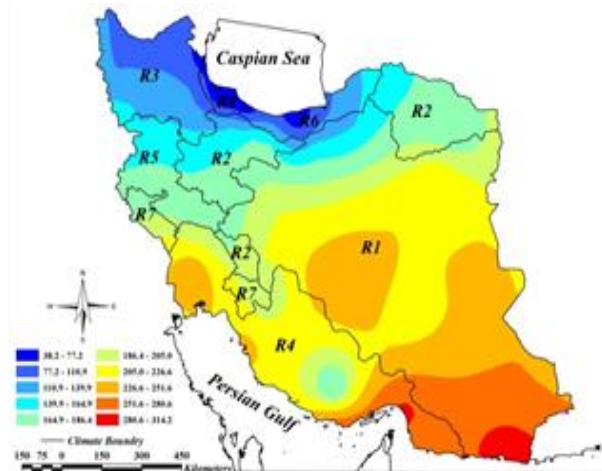
شکل ۲۳- نقشه ی حداکثر سالانه ی روز های بدون بارندگی در دوره ی برگشت ۱۰ ساله.
