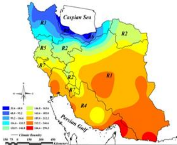
شکل ۲۰ نقشه ی حداکثر سالانه ی روزهای بدون بارندگی در دوره ی برگشت ۵ ساله.
