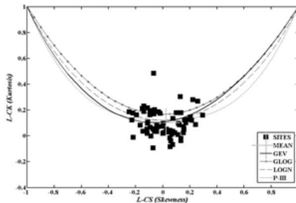
شکل ۹- نمودار نسبی مقادیر LCs در برابر LCK داده های روزهای بدون بارش.
