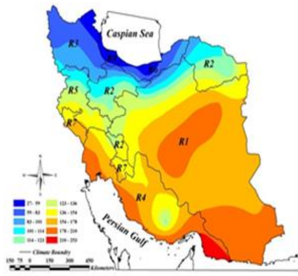
شکل ۲- میانگین تعداد روزهای بدون بارندگی در مناطق مختلف ایران.
