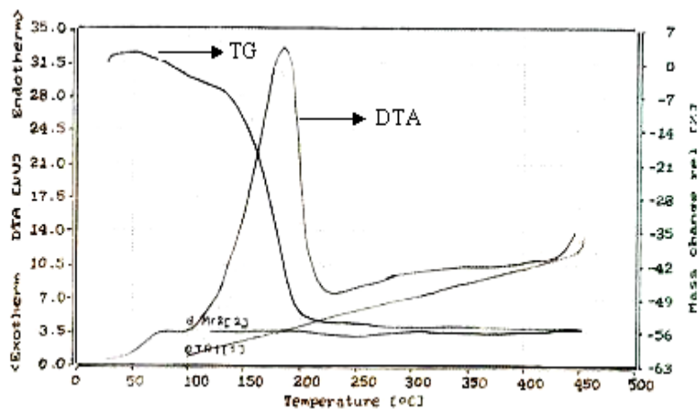
شکل ۵- نمودار DTA و TG گچ قالب سازی گچ بتا
