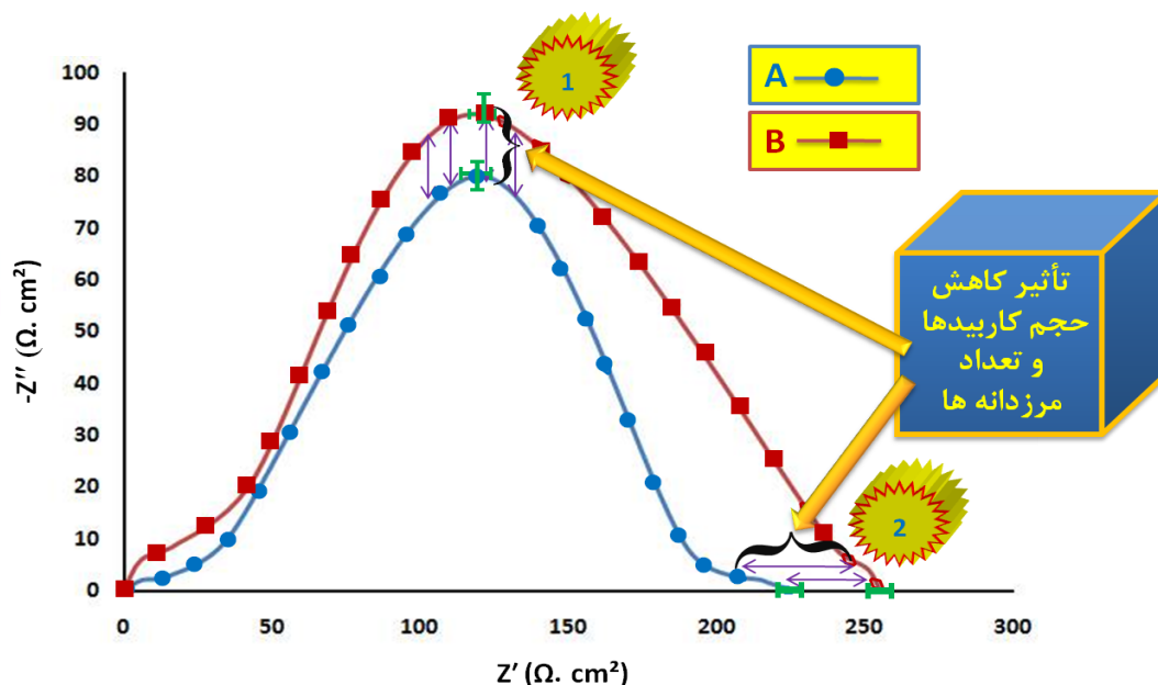
شکل ۶- نمودار نایکویست مربوط به آزمون طیف سنجی امپدانس الکتروشیمیایی در حداقل سه بار تکرارپذیری
