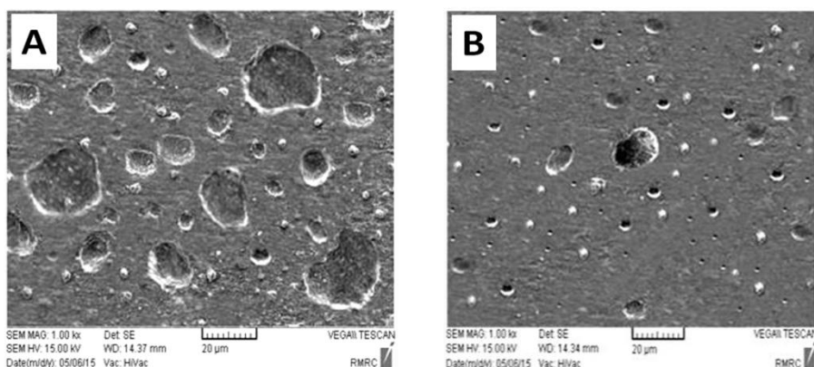
شکل ۷- تصاویر SEM از سطح مورد استفاده ی نمونه‌ها در آزمون‌های الکتروشیمیایی
