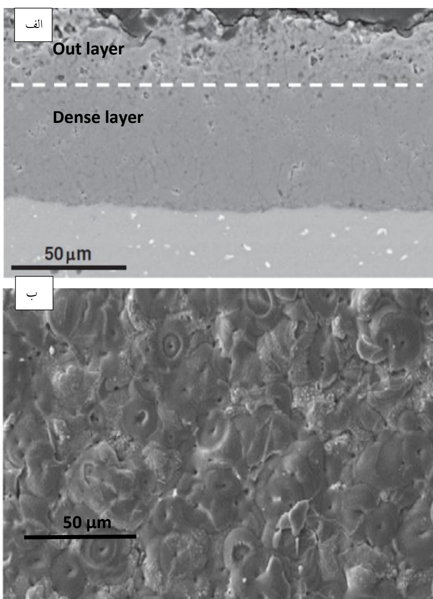
شکل ۵- الف) تصویر میکروسکوپ الکترونی روبشی از مقطع ب) تصویر میکروسکوپ الکترونی روبشی از سطح نمونه
