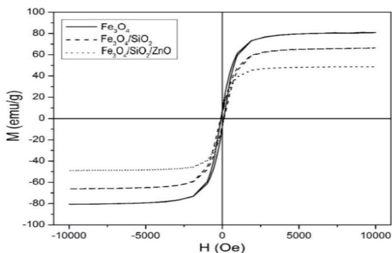
شکل ۸ - منحنی ویژگی‌های مغناطیسی برای ذرات \text{Fe}_3\text{O}_4 و نانوساختارهای \text{Fe}_3\text{O}_4/\text{SiO}_2 و \text{Fe}_3\text{O}_4/\text{SiO}_2/\text{ZnO} در
