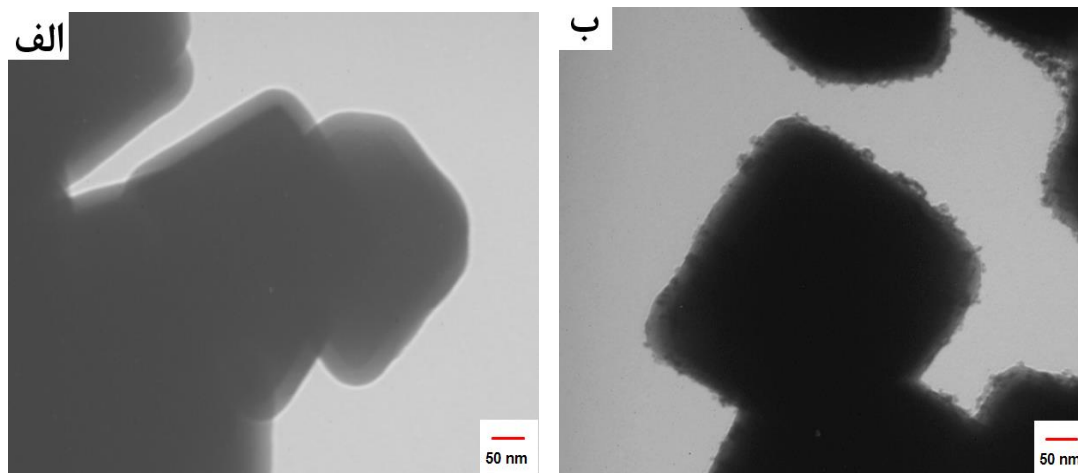
شکل ۵ - تصاویر TEM نانوساختارهای (الف) Fe_3O_4/SiO_2 و (ب) Fe_3O_4/SiO_2/ZnO با ساختار هسته/پوسته/پوسته
