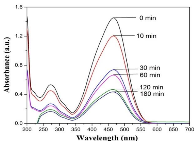
شکل ۱۰- منحنی های جذب محلول متیلن نارنجی (با غلظت اولیه ۱۰ میلی گرم بر لیتر) در زمان های متفاوت، تحت تابش نور
