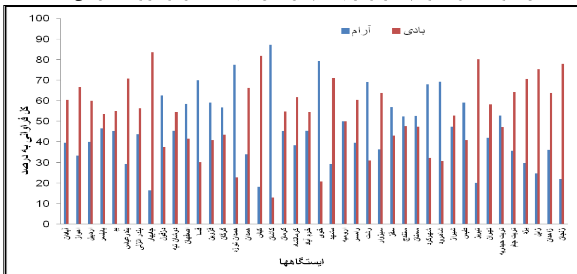
شکل ۳- مجموع سالانه درصد فراوانی دوره های بادی و دوره های همراه با شرایط آرام در ایستگاههای مورد مطالعه
