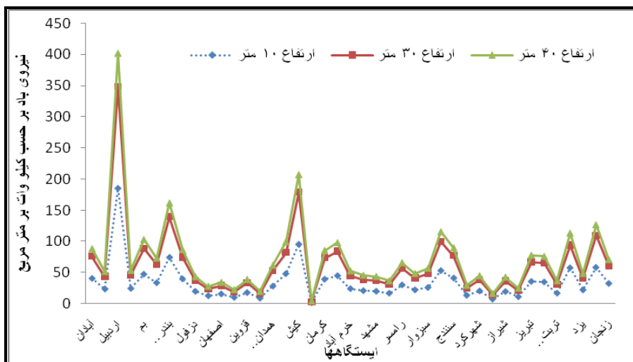
شکل ۱۱- توان چگالی بادی بر حسب وات بر متر مربع در فصل پاییز
