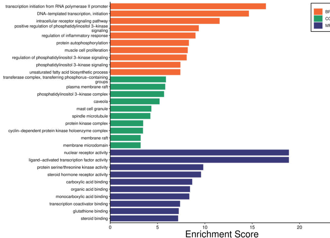
شکل ۴- بررسی آنتولوژی ژنی زن‌های مشترک بربرین در سرطان تخمدان به ترتیب در سه بخش BP, CC و MF.
