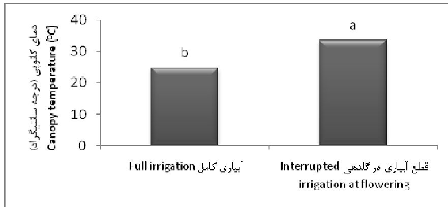
شکل ۶- اثر سطوح آبیاری بر دمای کانوپی Figure 6. Effect of irrigation levels on canopy temperature
