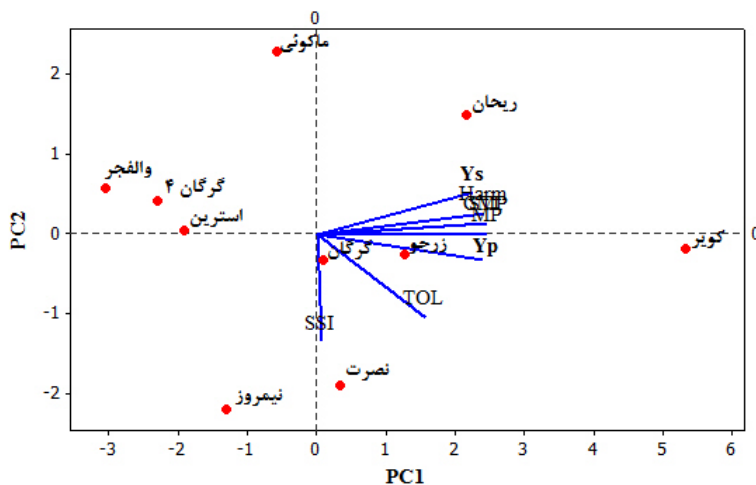
شکل ۱- نمودار بای پلات حاصل از تجزیه به مؤلفه‌های اصلی روی مقادیر شاخص‌های انتخاب برای ارقام جو مورد بررسی Figure 1. Biplot diagram obtained by principal component analysis on the values of selection indices for the studied barley cultivars
