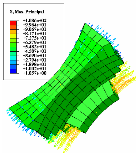
شکل (۸) بردارهای تنش ماکزیمم اصلی در اثر بارهای همبندی در پل بین دریچه‌های گاز و دود.
