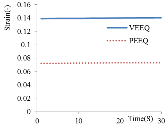
شکل (۱۷) نمودارهای کرنشهای پلاستیک معادل و ویسکوز معادل برای نقطه یک المان ۵۰۱۵۲
