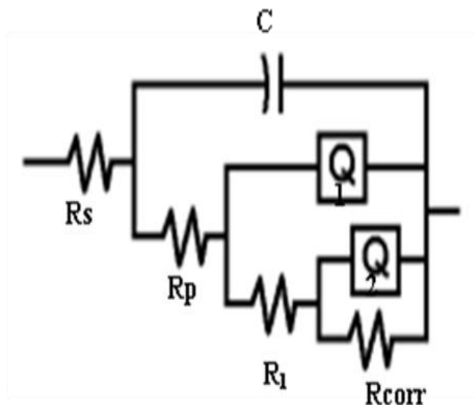
شکل (۶): مدار معادل پیشنهادی جهت مدل‌سازی داده‌های امپدانس برای نواحی مختلف جوش
