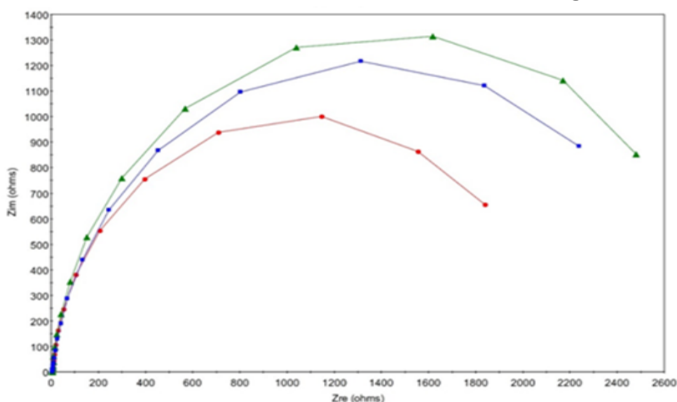
شکل (۵): منحنی های نایکوئیست نواحی مختلف جوش (●) فلز پایه، (■) ناحیه متاثر از جوش (HAZ)، (▲) ناحیه دکمه جوش (WNZ)
