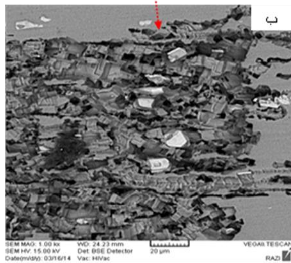
شکل (۱۰): تصاویر میکروسکوپ الکترونی روبشی (توسط الف): الکترون های ثانویه، (ب): برگشتی) از حفرات کریستالوگرافی (بلور شناسی) در ناحیه متاثر از جوش
