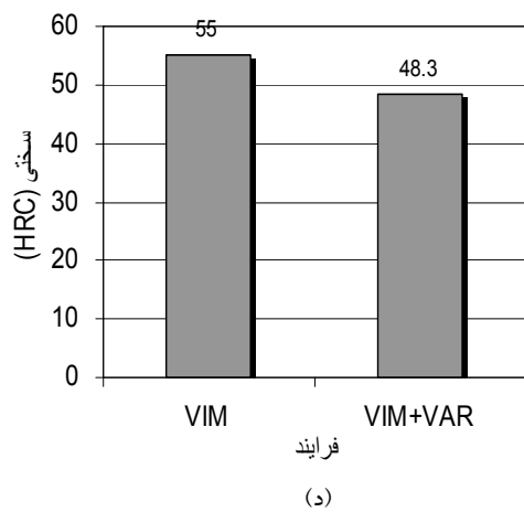
شکل (۳): تأثیر فرآیند VAR بر (الف) استحکام، (ب) انعطاف‌پذیری، (ج) مقاومت به ضربه و (د) سختی فولاد C۳۰۰ حاوی ۰/۶۵ درصد وزنی تیتانیم تولید شده به روش VIM.
