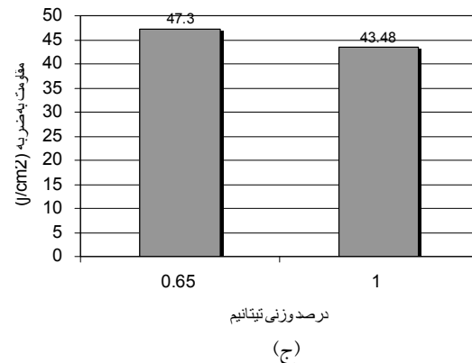
شکل (۶): مقایسه (الف) استحکام، (ب) انعطاف پذیری، (ج) مقاومت به ضربه و (د) سختی دو فولاد C۳۰۰ حاوی ۰/۶۵ و ۱ درصد وزنی تیتانیوم تولید شده به روش VIM + VAR.
