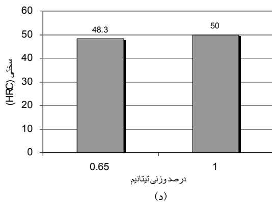
شکل (۶): مقایسه (الف) استحکام، (ب) انعطاف پذیری، (ج) مقاومت به ضربه و (د) سختی دو فولاد C۳۰۰ حاوی ۰/۶۵ و ۱ درصد وزنی تیتانیوم تولید شده به روش VIM + VAR.
