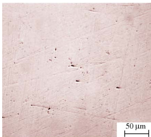
شکل (۴): شمایی از مقدار، اندازه و توزیع آخال‌های موجود در شمش ریخته‌گری شده با روش‌های (الف) VIM و (ب) VIM+VAR.
