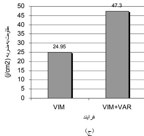
شکل (۳): تأثیر فرآیند VAR بر (الف) استحکام، (ب) انعطاف‌پذیری، (ج) مقاومت به ضربه و (د) سختی فولاد C۳۰۰ حاوی ۰/۶۵ درصد وزنی تیتانیم تولید شده به روش VIM.
