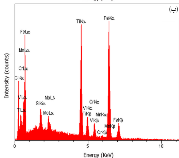
شکل (۸): نتایج طیف سنجی EDS: (الف): فاز زمینه و (ب): ذره صلیبی در نمونه آلیاژسازی شده با لایه پیش‌نشاندن شده 50 \mu\text{m}
