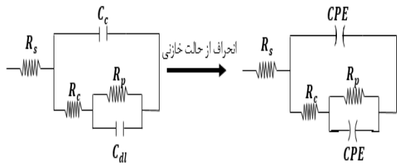
شکل (۱): مدار معادل آرماتور فولادی در بتن با مقاومت بالا
