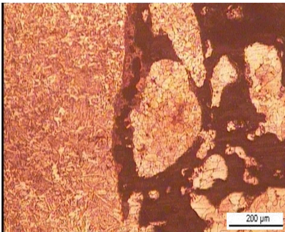
شکل (۷): نمونه ترمیم یافته با اندازه دهانه شیار برابر با 1 میلیمتر، عیوب متالورژیکی به رنگ تیره در محل ترمیم یافته، میکروسکپ نوری شرکت Dewinter، روش جوشکاری شعله‌ای با پاشش
