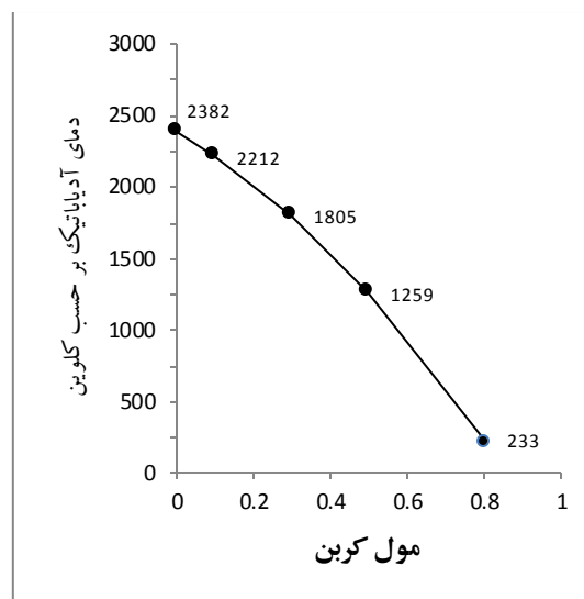
شکل (۳): نمودار تغییر دمای آدیباتیک واکنش احیا همزمان اکسید مس با کربن و روی بر حسب افزایش میزان مول کربن
