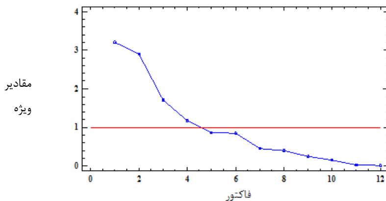
شکل ۱- نمودار اسکری گراف برای تعیین تعداد عامل‌ها
