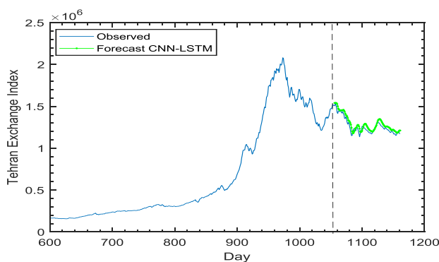
شکل (۶). پیش‌بینی شاخص بورس اوراق بهادار تهران بر اساس مدل CNN-
