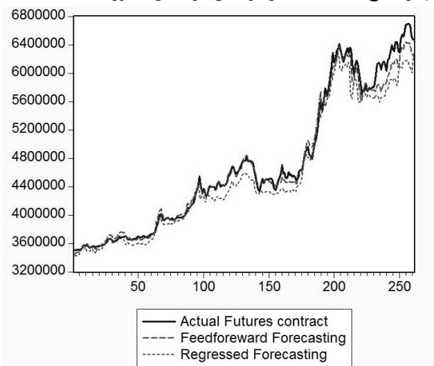
شکل ۵. مقایسه مقدار های پیش‌بینی شده شبکه عصبی و رگرسیون خطی با مقادیر واقعی در
