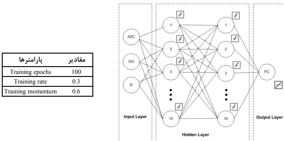
شکل ۲. شبکه عصبی طراحی شده در این تحقیق
